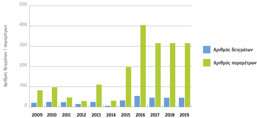
Σχήμα 36: Διαχρονική παρουσίαση ελέγχου δειγμάτων πόσιμου νερού για ραδιονουκλίδια (2009-2019)
